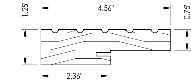
1 WOOD JAMB
