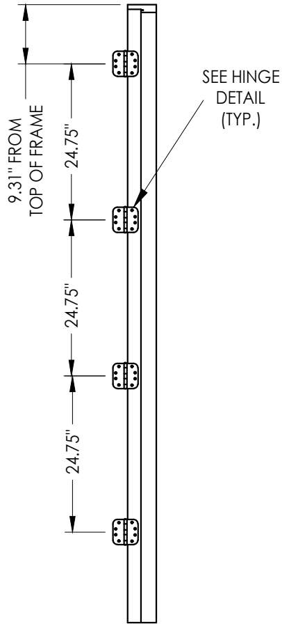
HINGE JAMB
